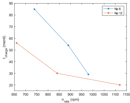
Gambar 7. Grafik Pengaruh Kecepatan Putaran Roda Rata Rata dan Jumlah Kutub terhadap Waktu Pengisian Aki
