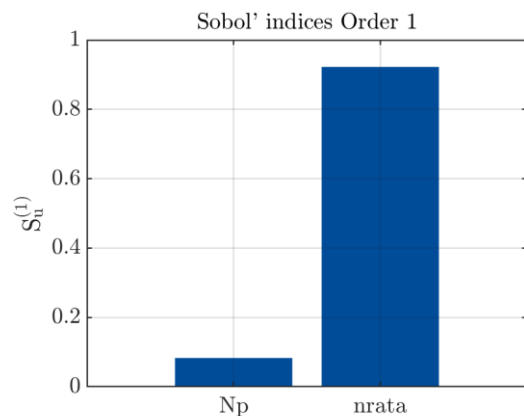
Gambar 6. Indeks Sensitivitas dari Masing-Masing Variabel Bebas
