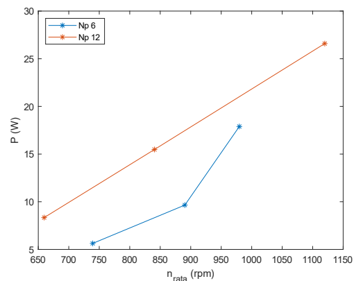
Gambar 5. Grafik Pengaruh Kecepatan Putaran Roda Rata Rata dan Jumlah Kutub terhadap Daya Listrik
