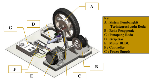
Gambar 3. Desain Setup Eksperimen Penelitian
