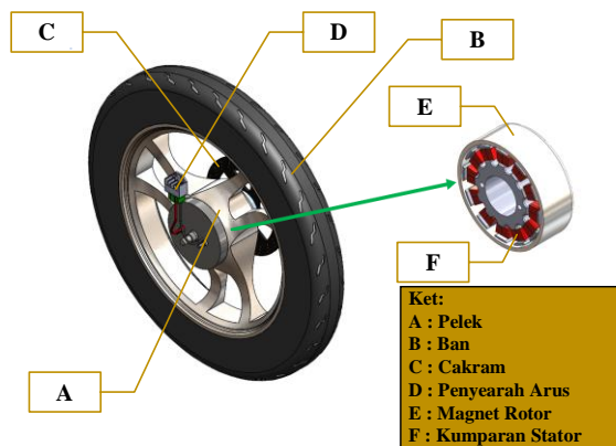
Gambar 1. Desain Prototipe Sistem Pembangkit Daya Listrik Terintegrasi pada Roda Kendaraan
