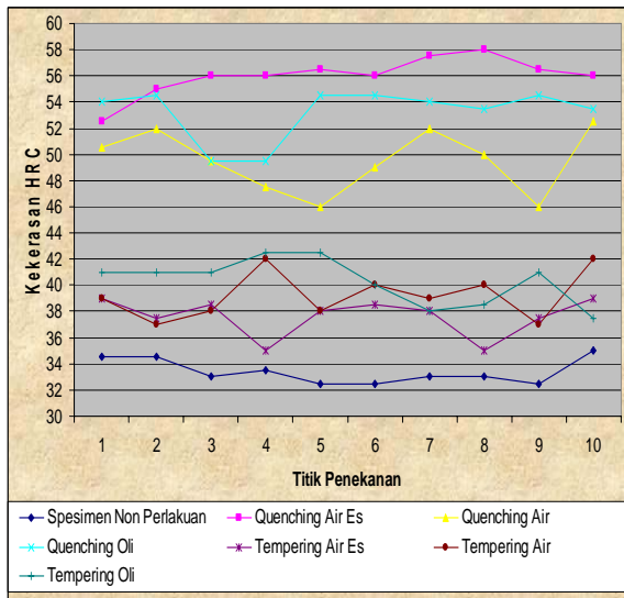
Gambar 6. Kurva Kekerasan Spesimen Non Perlakuan, Spesimen Yang Diquench Dan Spesimen Yang Diquench dan Ditemper Dengan Media Pendingin berbeda.
